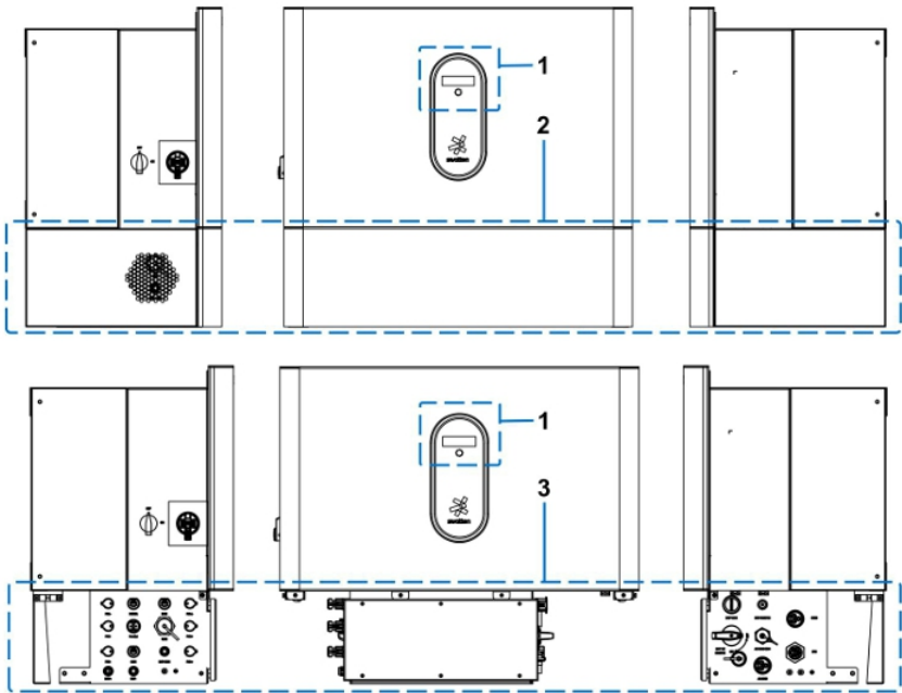
Figura 2-1 Aspetto dell'inverter
