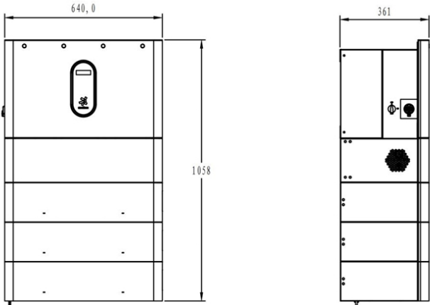
Figura 2-2 Dimensioni dell'inverter
