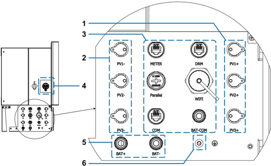
Figura 6-1 Terminali
