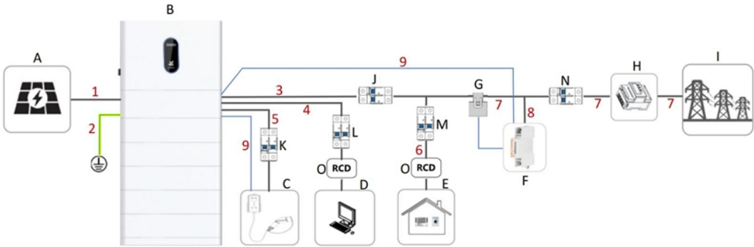
Diagramma di cablaggio del sistema
