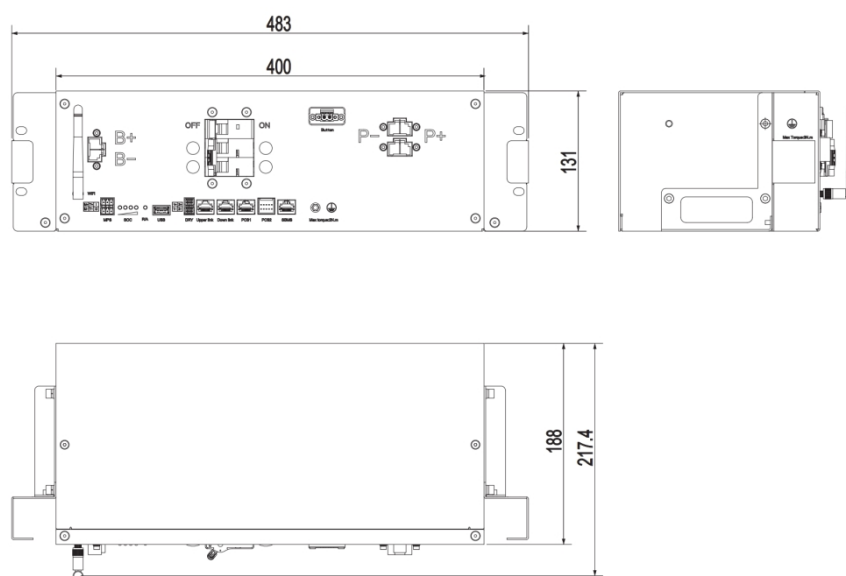
Figura 2-3 Modulo
