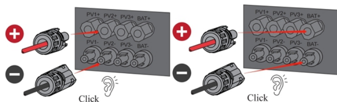
(1) Collegamento dei cavi FV
