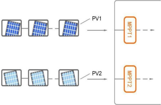
Figura 6-3 Configurazione degli ingressi fotovoltaici
