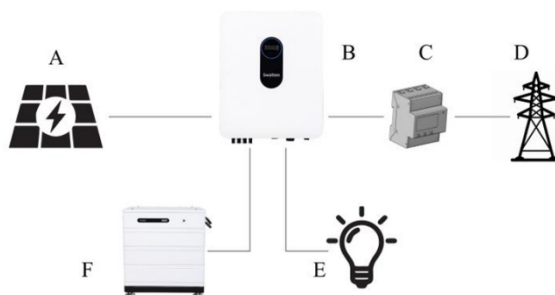
Figura 2-4 Sistema di accumulo dell'energia fotovoltaica
