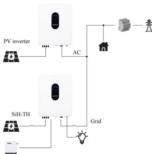
Figura 2-9 Porta On-grid per il retrofitting del sistema fotovoltaico esistente
