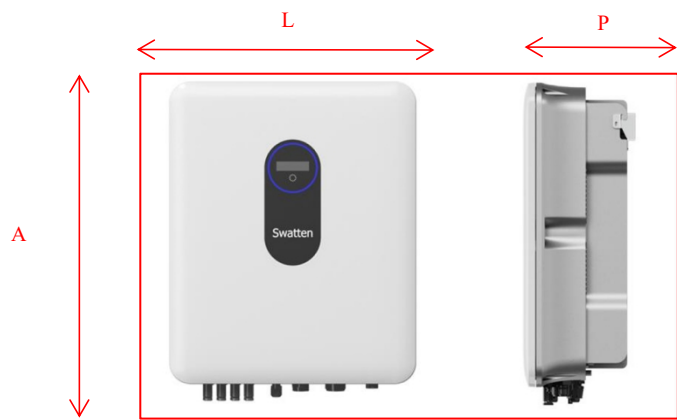
Figura 2-2 Dimensioni dell’inverter
