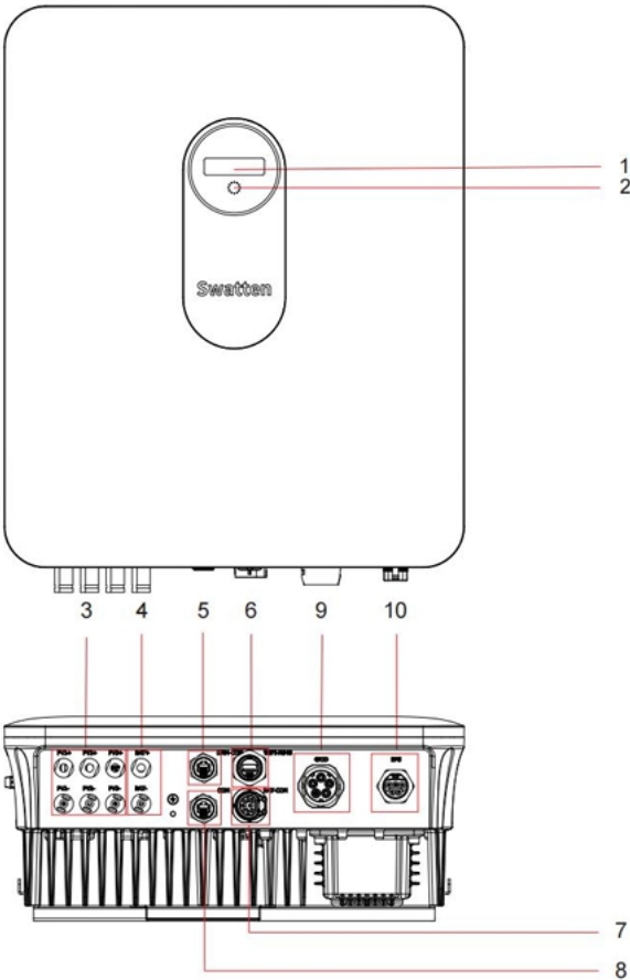
Figura 6-1 Terminali
